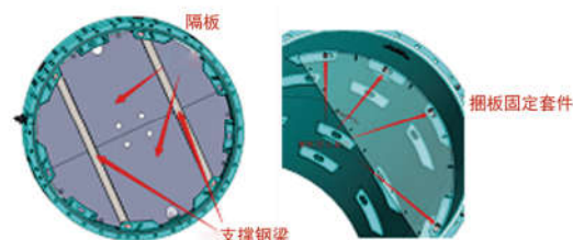
安装底层隔板
